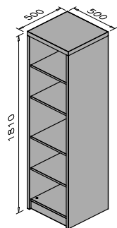
87087 Armário charuto sem portas
