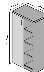
87067E Armário alto com 1 porta de giro no lado esquerdo
