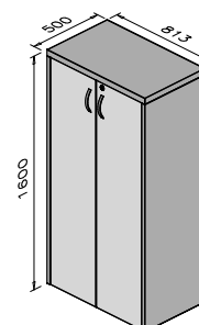
87067 Armário alto fechado com portas de giro
