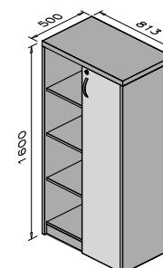
87067D Armário alto com 1 porta de giro no lado direito
