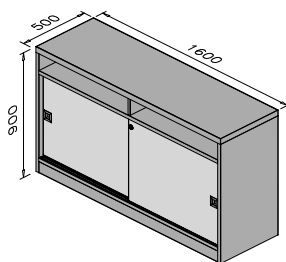
87077CO Armário aparador com portas de correr e nichos superiores
