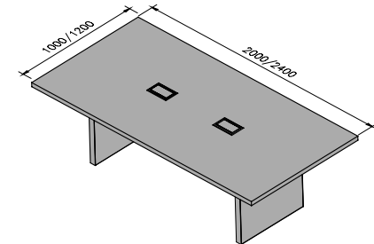
87200 / 87240 Mesa de Reunião com caixas de tomada e calha eletrificável sob o tampo
