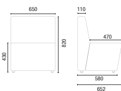
36.865 Módulo Reto 650mm
