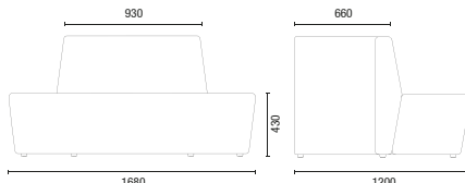
36.890 IN Módulo Curvo Encosto Interno 90°
