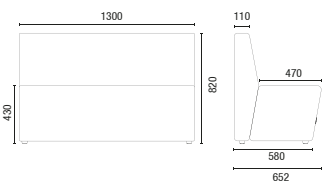
36.813 Módulo Reto 1300mm
