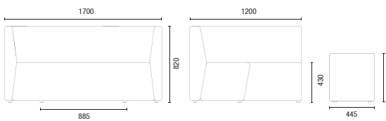
36.890 EX Módulo Curvo Encosto Externo 90°
