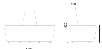
36.818 Módulo Ponta Encosto Interno 180°
